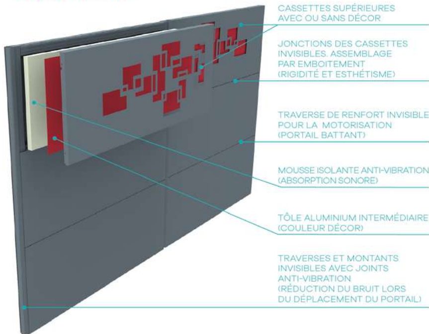
THERMOLAQUÉ RAL 7016
