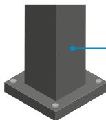
POTEAU TUBULAIRE AVEC PLATINE DE FIXATION AU SOL DÉBORDANTE Poteau 125 x 125 pour la descente des eaux pluviales. Platine visible débordante. 190 x 190 mm.
