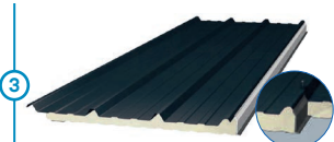
PANNEAU ACIER GALVANISÉ ET ISOLÉ ONDULATION 85 MM Face supérieure laquée gris RAL 7016, blanc RAL 9010 ou tuile RAL 8012. Face inférieure laquée blanc. Mousse isolante 40 mm. Panneau de 1 000 mm x 5 000 mm maxi. Hauteur ondulation de 85 mm. Poutre intermédiaire à partir d'une avancée de 4 000 mm.
