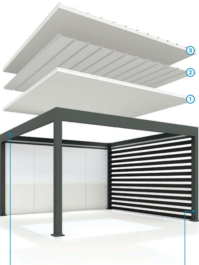
POUTRE 246 X 47 MM À l'avant, chéneau pour l'évacuation des eaux de pluie.
