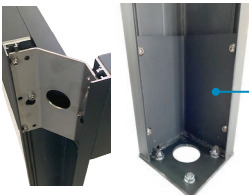
POTEAU RECONSTITUÉ AVEC PLATINE DE FIXATION AU SOL INVISIBLE Poteau reconstitué avec renfort 125 x 125 pour la descente des eaux pluviales. Platine invisible. 125 x 125 mm.
