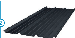
PANNEAU ACIER GALVANISÉ ONDULATION 39 MM Face supérieure laquée gris RAL 7016, blanc RAL 9010 ou tuile RAL 8012. Face inférieure laquée blanc. Panneau de 1 000 mm x 5 000 mm maxi. Au choix, avec ou sans feutre anti-condensation. Hauteur ondulation de 39 mm. Poutre intermédiaire à partir d'une avancée de 4 000 mm.
